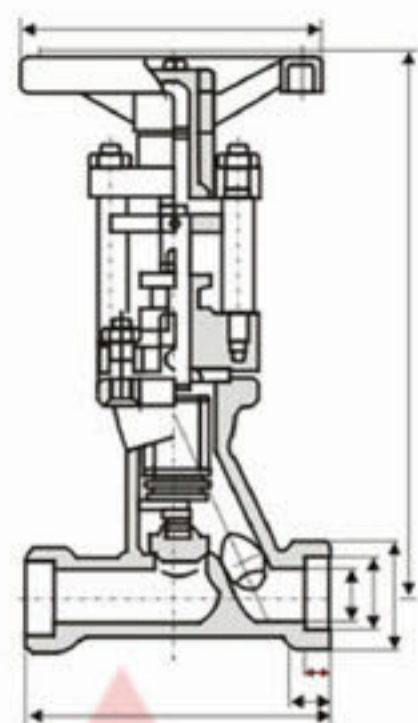
主要外形和连接尺寸 Main External and Connection Dimension(WJ61)
